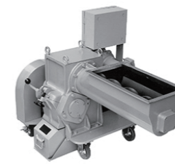
機 械 名 / PS-180 モーター / 6P 1.5kW 機械寸法 / 1,240mm (W) 810mm (L) 955mm (H) 機械重量 / 410kg
