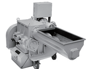
機 械 名 / PS-360 モーター / 6P 2.2kW 機械寸法 / 1,580mm (W) 815mm (L) 1,035mm (H) 機械重量 / 530 kg
